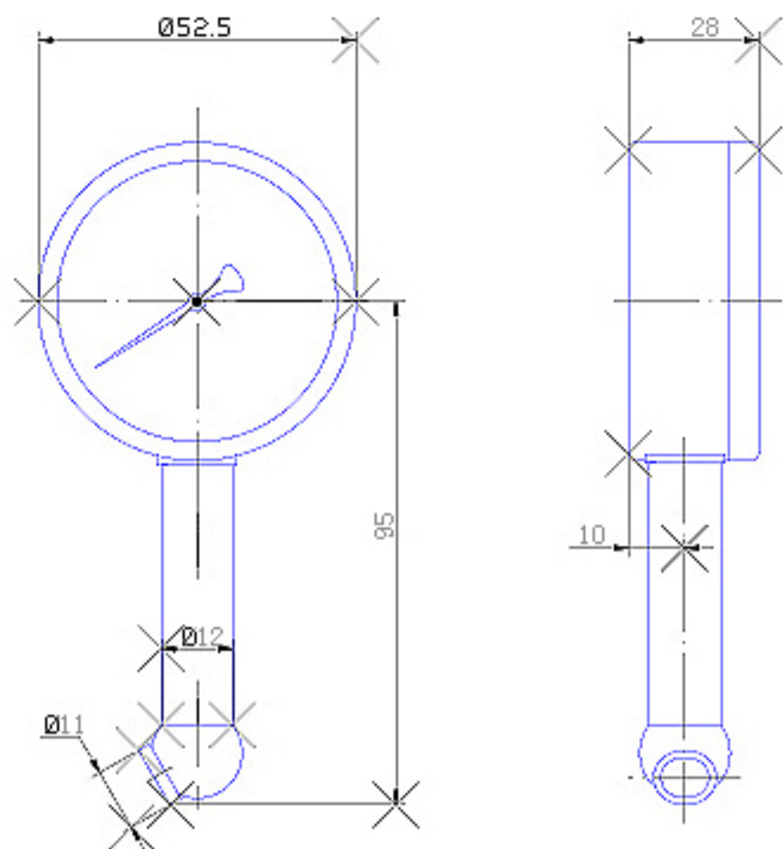
Y-2" 轮胎表 (一)
